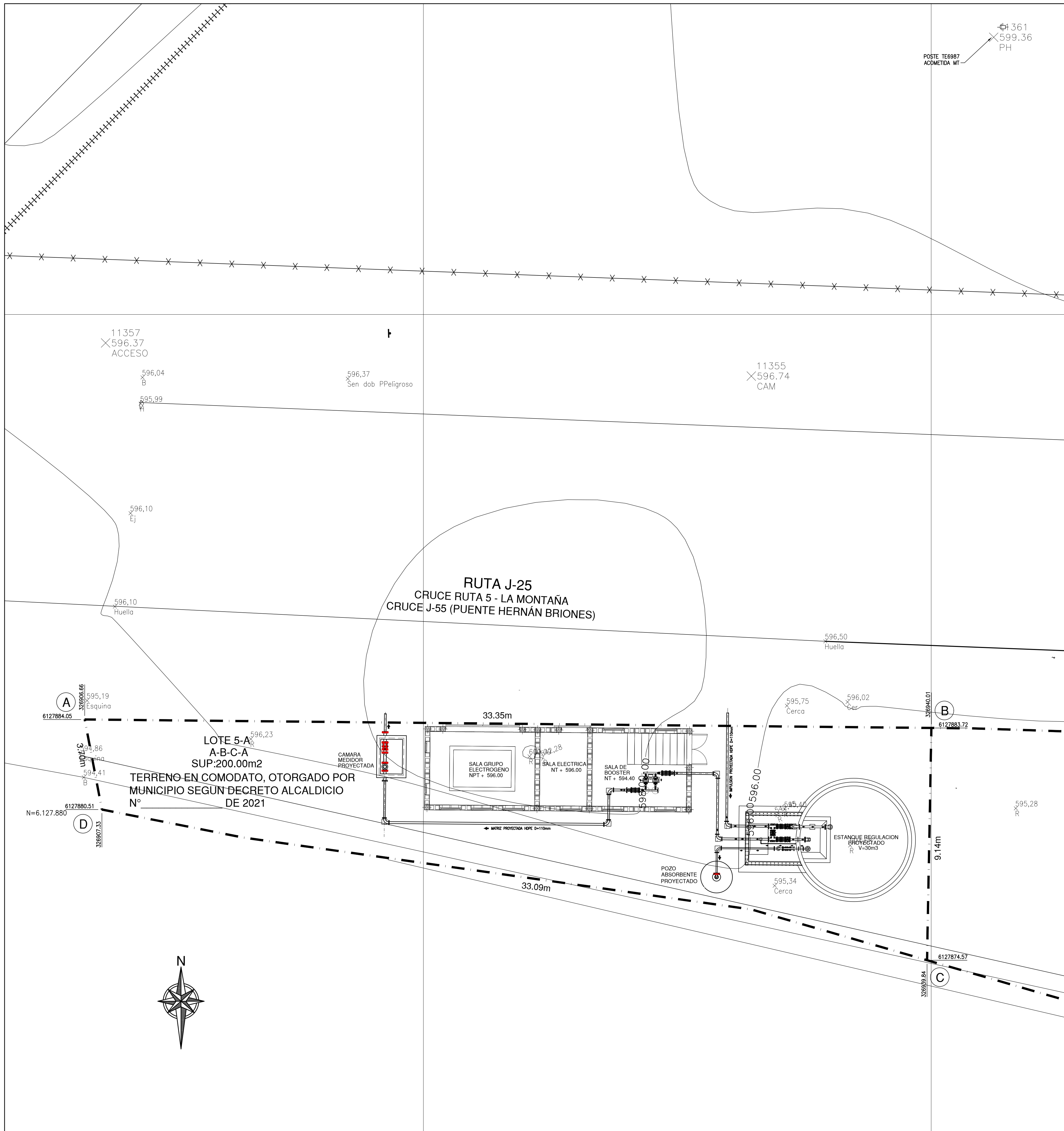
PLANTA RECINTO RELEVACION N°2 ESCALA 1:75
